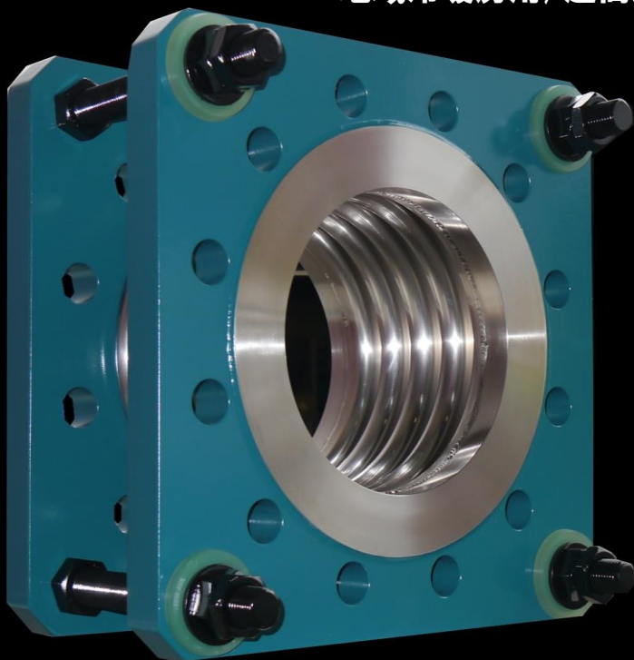
IW830 (3MPa) 200A x 230L
