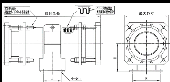
JIS B2352 A型 複式 3MPaタイプ
