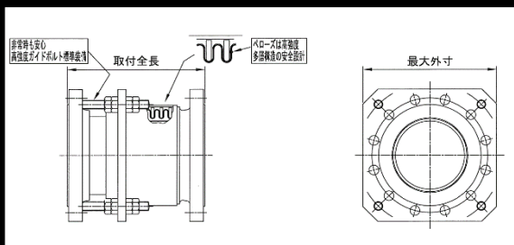
JIS B2352 A型 単式 3MPaタイプ
